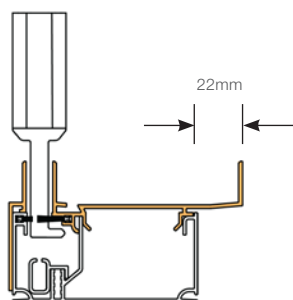
S4 Unsichtbare Schwelle (mit 22mm Überstand)
