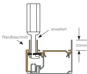
S4 Unsichtbare Schwelle
