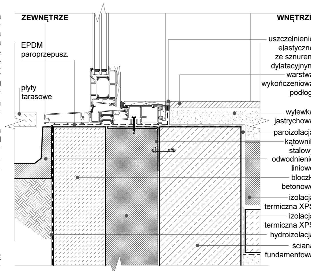
3 detal progu - poziom terenu
