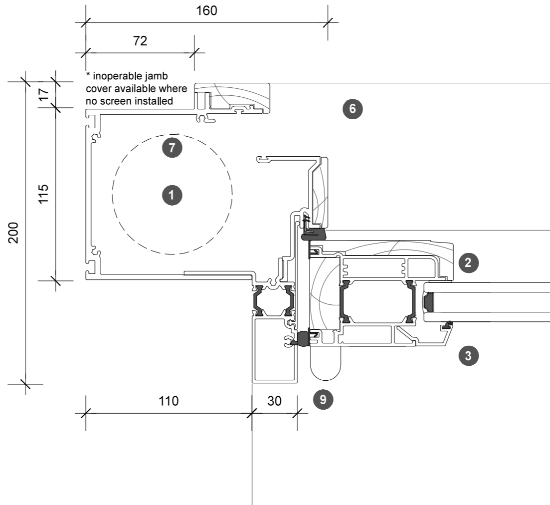
1. jamb detail
